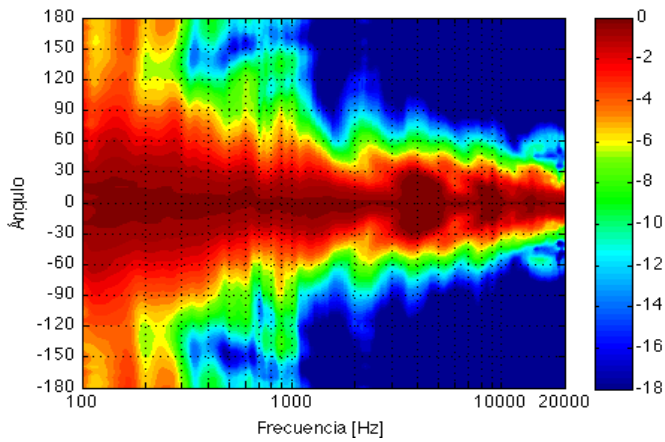
Directividad Vertical
