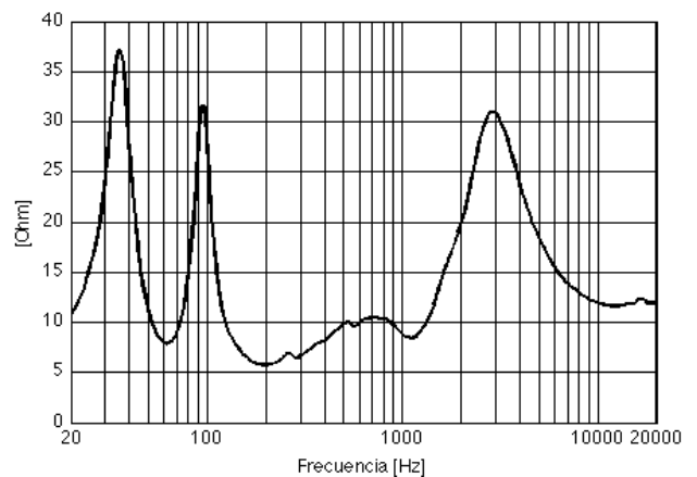
Impedancia
