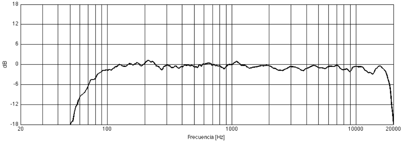
Directividad Horizontal
