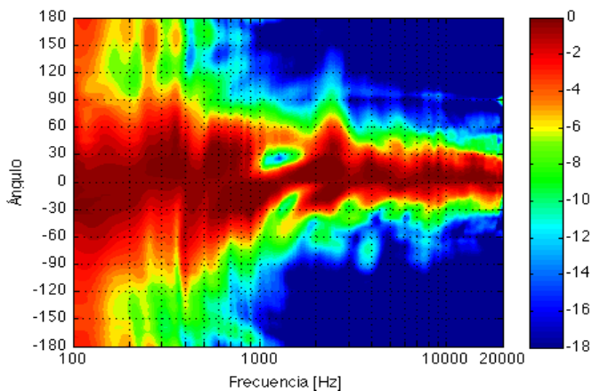
Directividad Vertical
