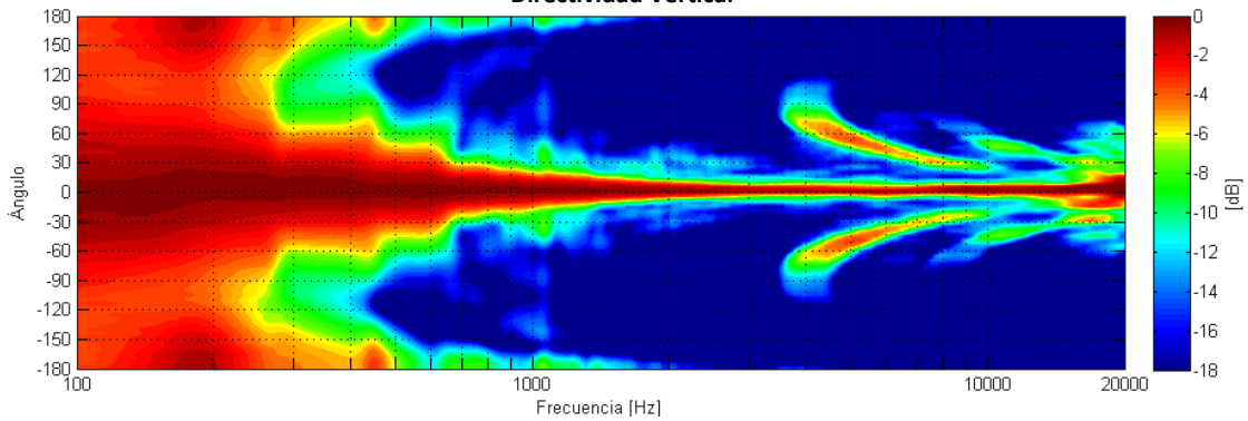
Directividad Vertical
