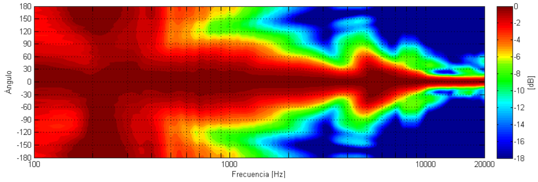
Directividad Horizontal
