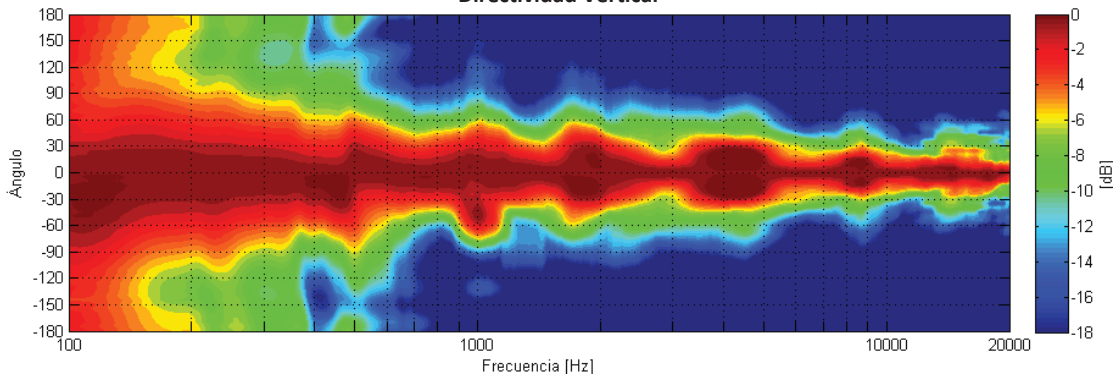
Directividad Vertical
