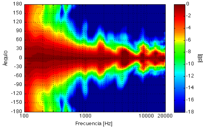
Directividad Vertical
