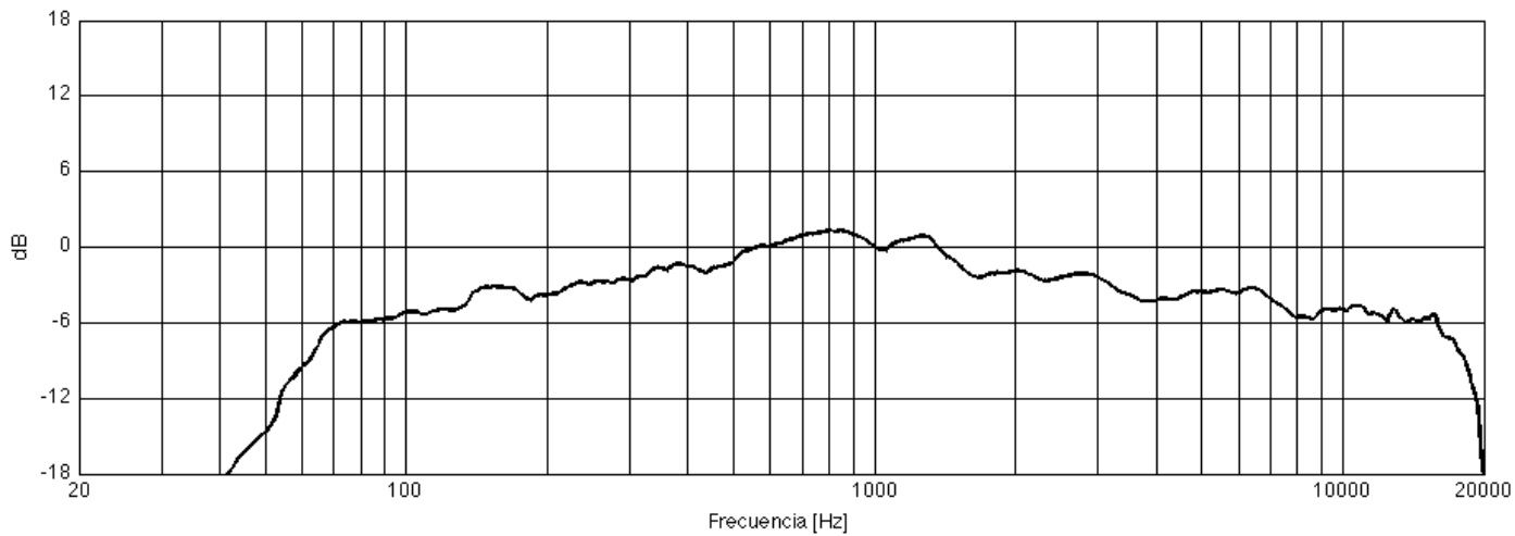
Directividad Horizontal
