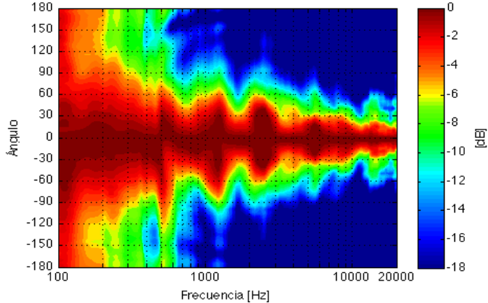
Directividad Vertical
