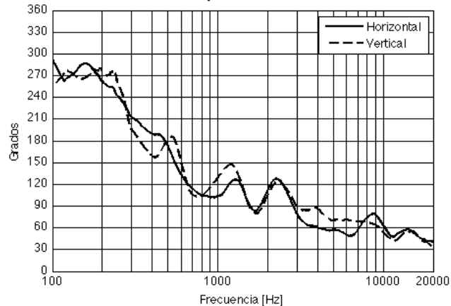
Dispersión a -6 dB
