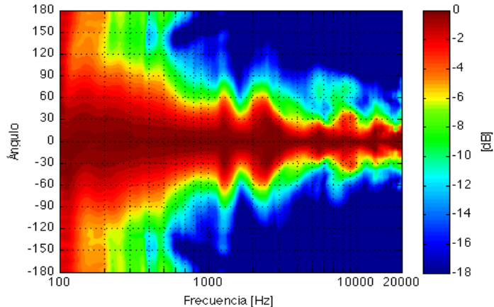
Directividad Horizontal
