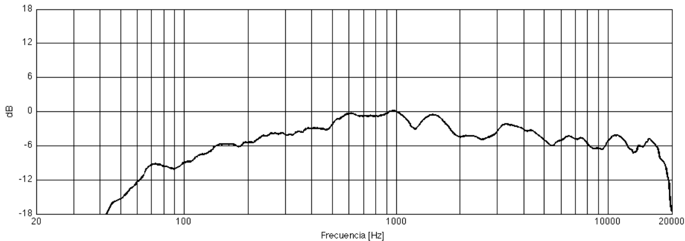
Directividad Horizontal
