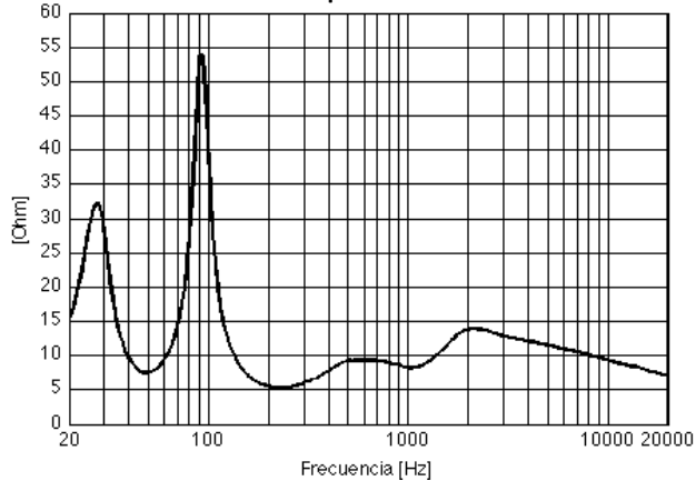
Impedancia
